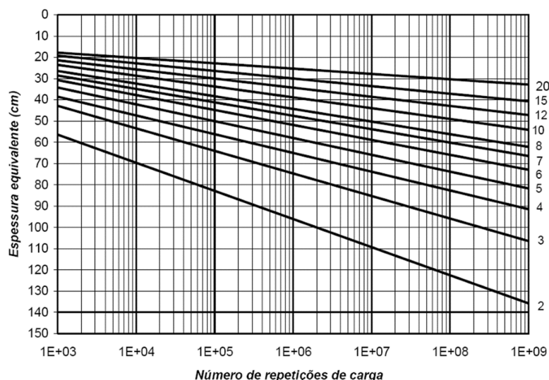
Figura 2 - Ábaco de dimensionamento
