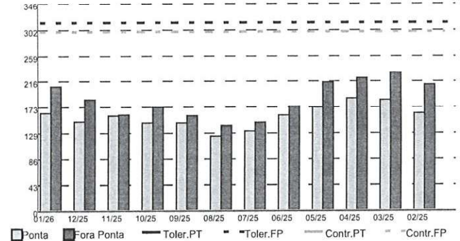
Demanda (kW)
